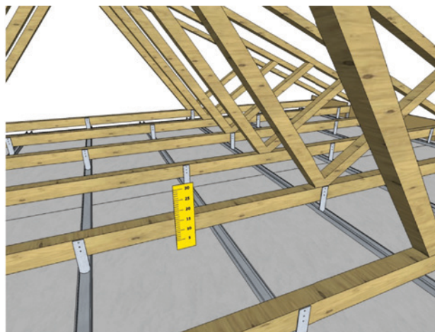
Figure 7 – Repérage de la hauteur d'isolant à souffler
